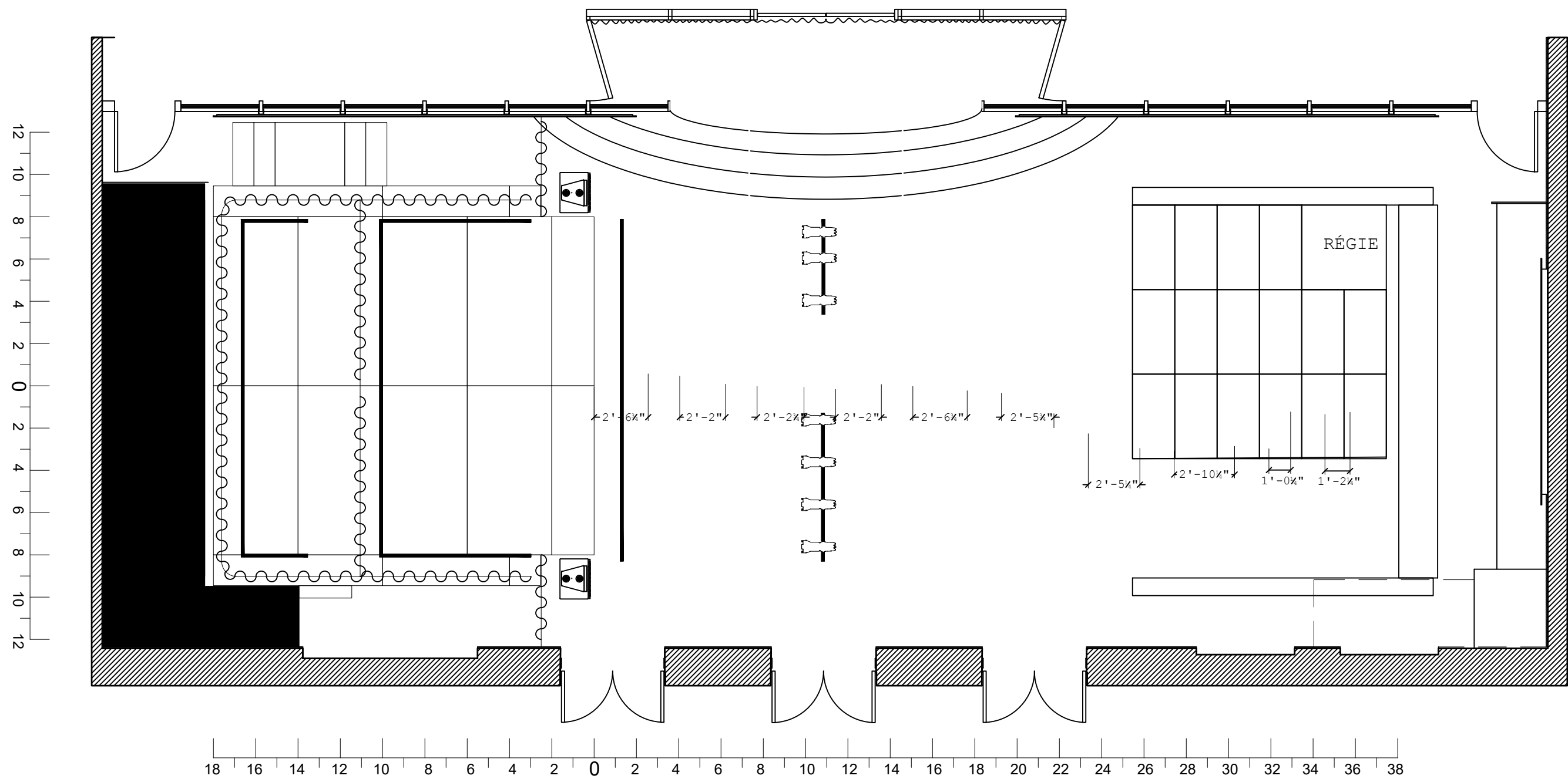
2 / 2 Vue en plan 3/16"=1'-0"
